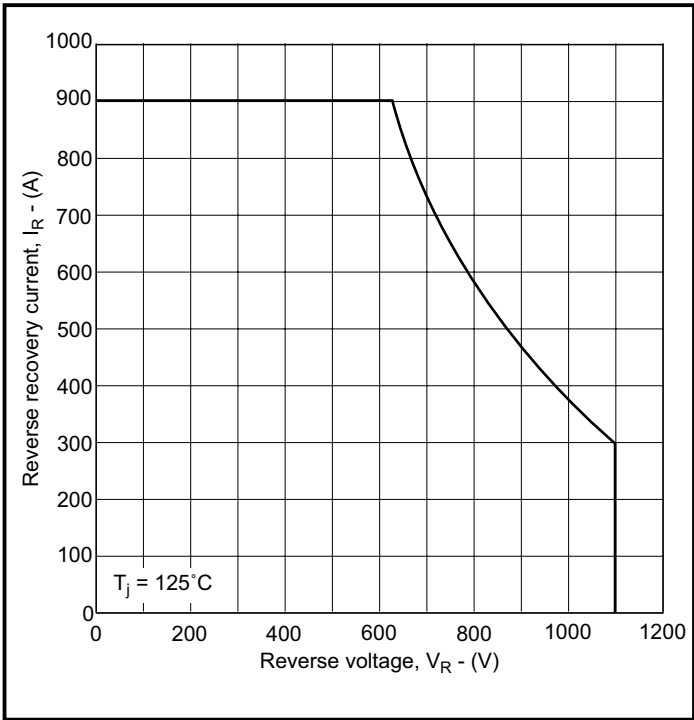
Fig. 7 RBSOA
