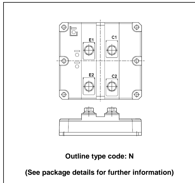
Fig. 2 Package
