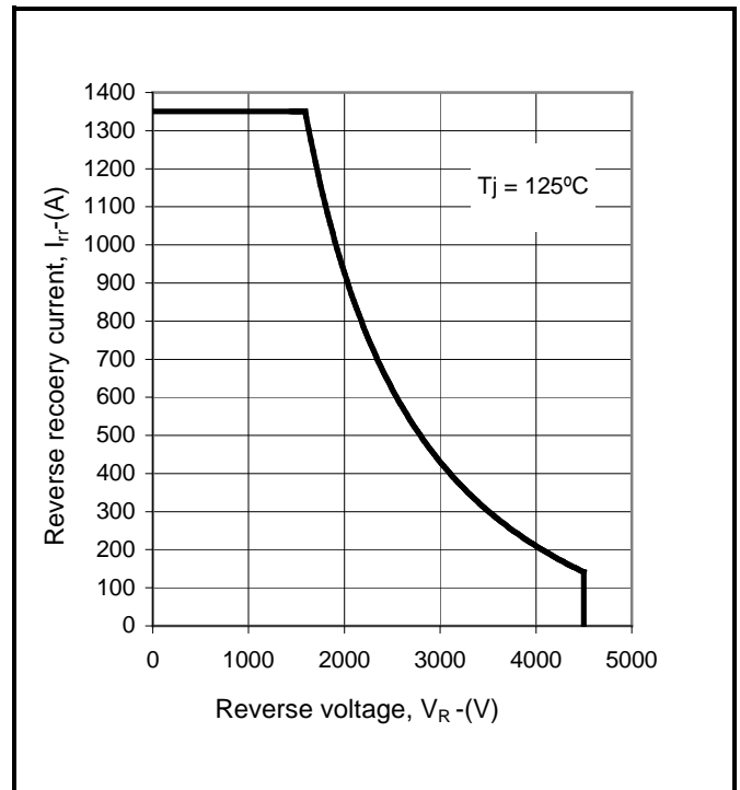
Fig.6 RBSOA
